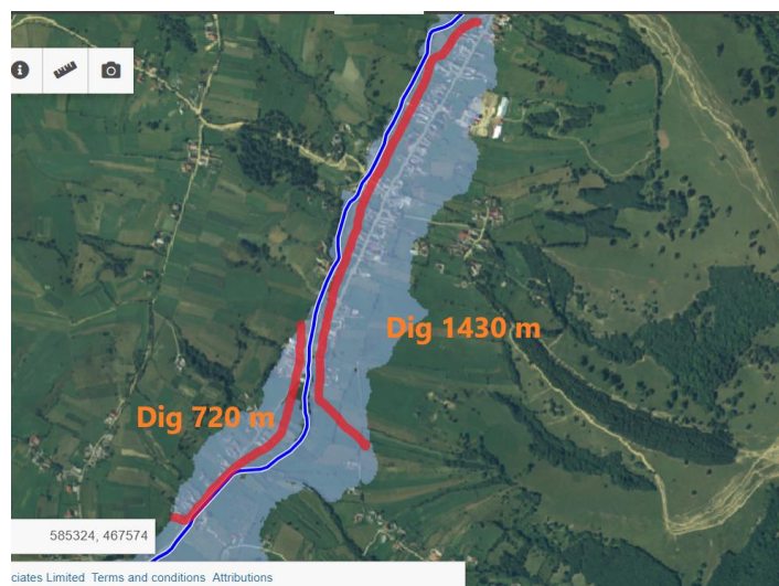
Diguri Barcani aval
