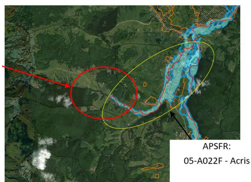
Acumularea nepermanentă Acriș – locația 1 V_{\text{reservoir}} = 3 \text{ mil. m}^3 H_{\text{dam}} = 25 \text{ m}
