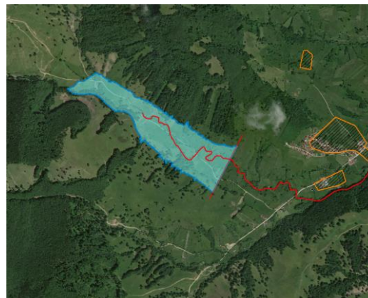
Acumularea nepermanentă Acriș – locația 1 V_{\text{reservoir}} = 3 \text{ mil. m}^3 H_{\text{dam}} = 25 \text{ m}
