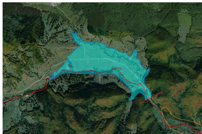
Acumularea nepermanentă Dălghiu, amonte de confluența cu râul Buzau V_{\text{reservoir}} = 9.5 \text{ mil. m}^3 H_{\text{dam}} = 30 \text{ m} 2 km de drum communal posibil de relocat
