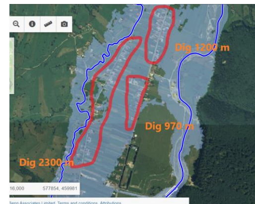
Diguri Acriș aval derivația Acriș-Buzău
