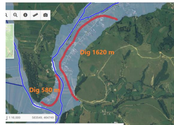
Diguri Lădăuți aval confluența Barcani
