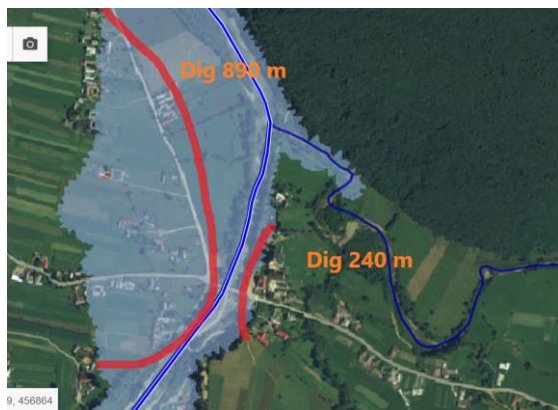
Diguri Buzău amonte confluența cu Pârâul de Câmp
