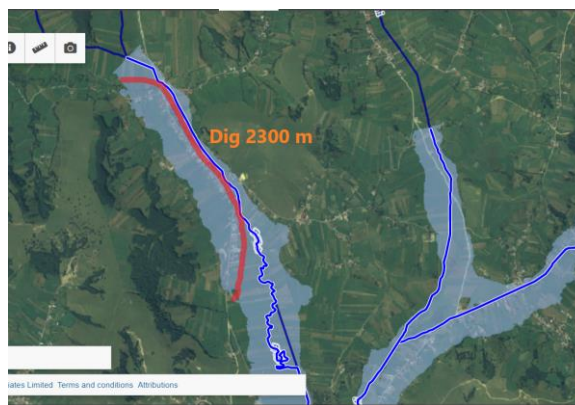
Dig râul Bârbat – localitatea Sărămaș
