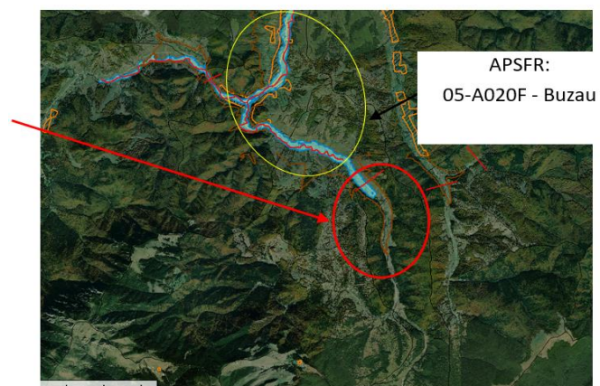
Acumularea nepermanentă Buzău, amonte de confluența cu afluentul Dălghiu V_{\text{reservoir}} = 7 \text{ mil. m}^3 H_{\text{dam}} = 30 \text{ m}
