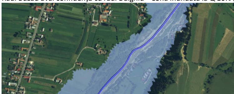
Râul Buzău aval confluența cu râul Dalghiu – zona inundată la Q 10% și Q 1%.
