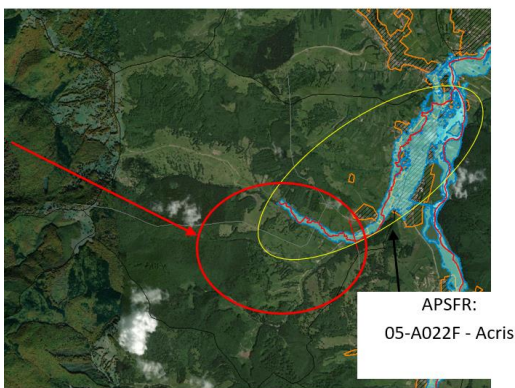
Acumularea nepermanentă Acriș – locația 2 V_{\text{reservoir}} = 9 \text{ mil. m}^3 H_{\text{dam}} = 30 \text{ m} Aproximativ 10 case de relocat
