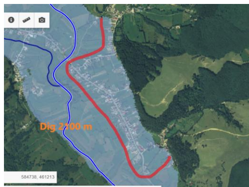
Diguri Buzău confluența Ciumernic
