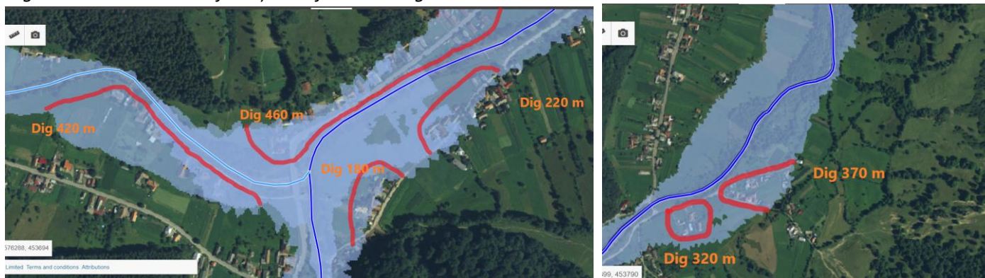
Diguri Buzău și Dălghiu amonte și aval de confluența
