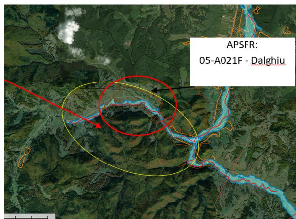
Acumularea nepermanentă Dălghiu, amonte de confluența cu râul Buzau V_{\text{reservoir}} = 9.5 \text{ mil. m}^3 H_{\text{dam}} = 30 \text{ m} 2 km de drum communal posibil de relocat
