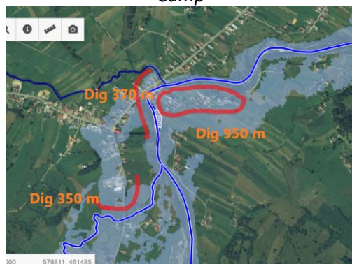
Diguri Buzău amonte -aval confluența Afiniș
