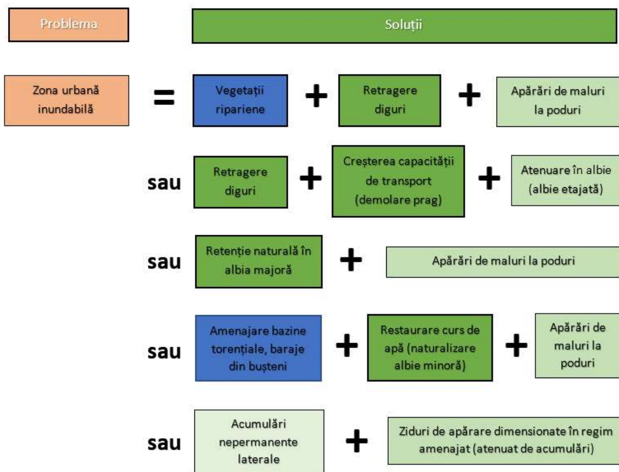
Figura 1. Reprezentare schematică a potențialelor abordări verzi, gri-verzi, gri
