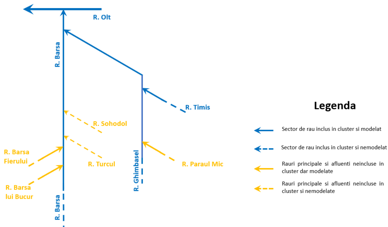
Figura 2: Schema sinoptică a proiectului
