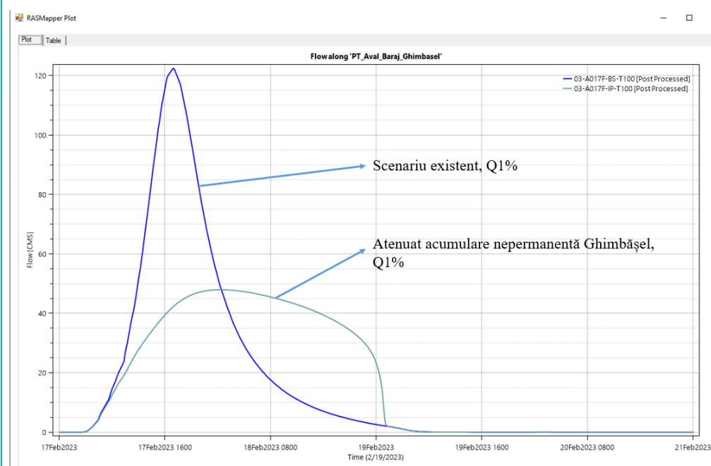
Figura 5: Hidrograful de debit pentru R. Ghimbășel în regim natural și hidrograful de debit defluent în urma realizării acumulării
