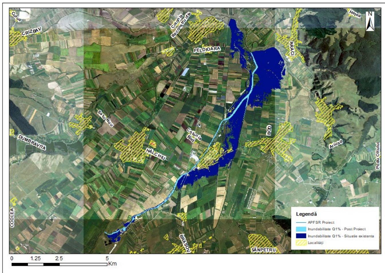
Figura 7: Limita de inundabilitate pre și post implementare proiect Q1% - r. Bârsa - 03-A015F
