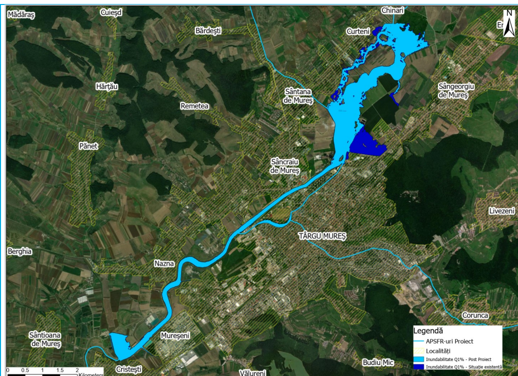
Figura 41: 2Limita de inundabilitate pre și post implementare proiect Q1%
