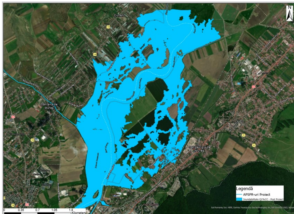
Figura 3: Limita de inundabilitate post implementare proiect Q1%+Schimbări climatice
