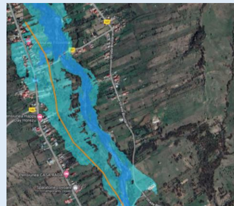
Diguri mal drept L = 1,3 \text{ km} , h = 1,5 \text{ m} loc. Romanii de Jos
