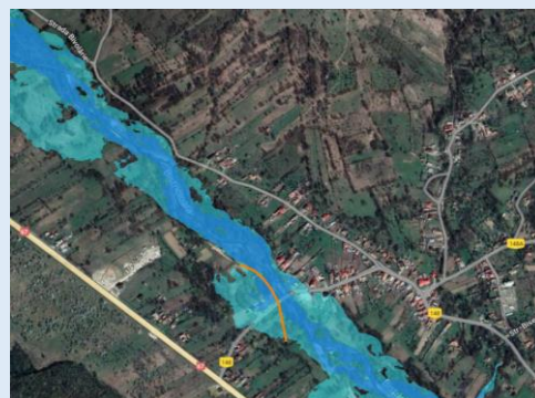
Diguri amonte si aval de pod DC 148 L = 0,3 \text{ km} , h = 1,5 \text{ m} , loc. Bogdanesti
