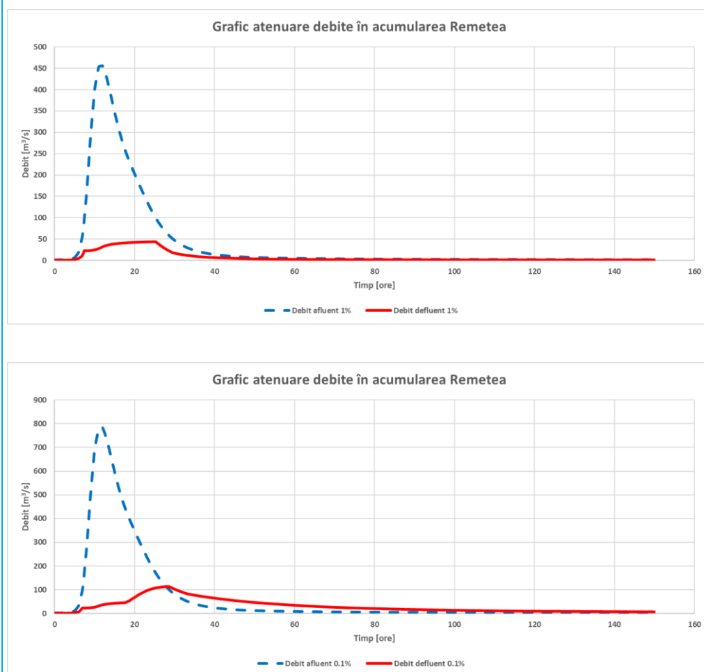
Figura 4- Graficul de atenuare în acumularea Remetea la 1% și 0,1%
