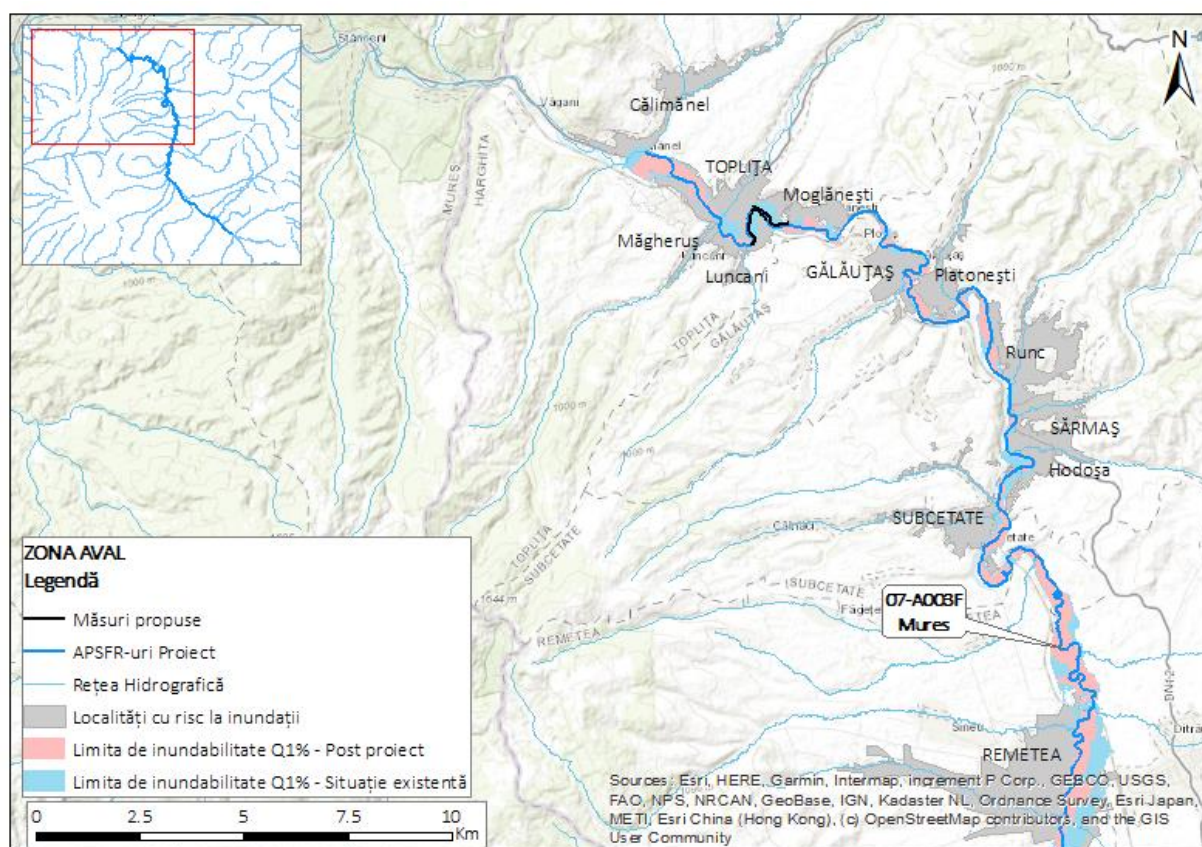
Figura 6: Limita de inundabilitate pre și post implementare proiect Q1%. Zona aval
