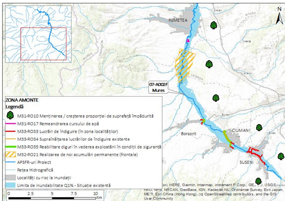
Figura 2: Localizarea măsurilor aferente alternativei preferate și limita de inundabilitate pentru probabilitatea de 1% în situația actuală. Zona amonte
