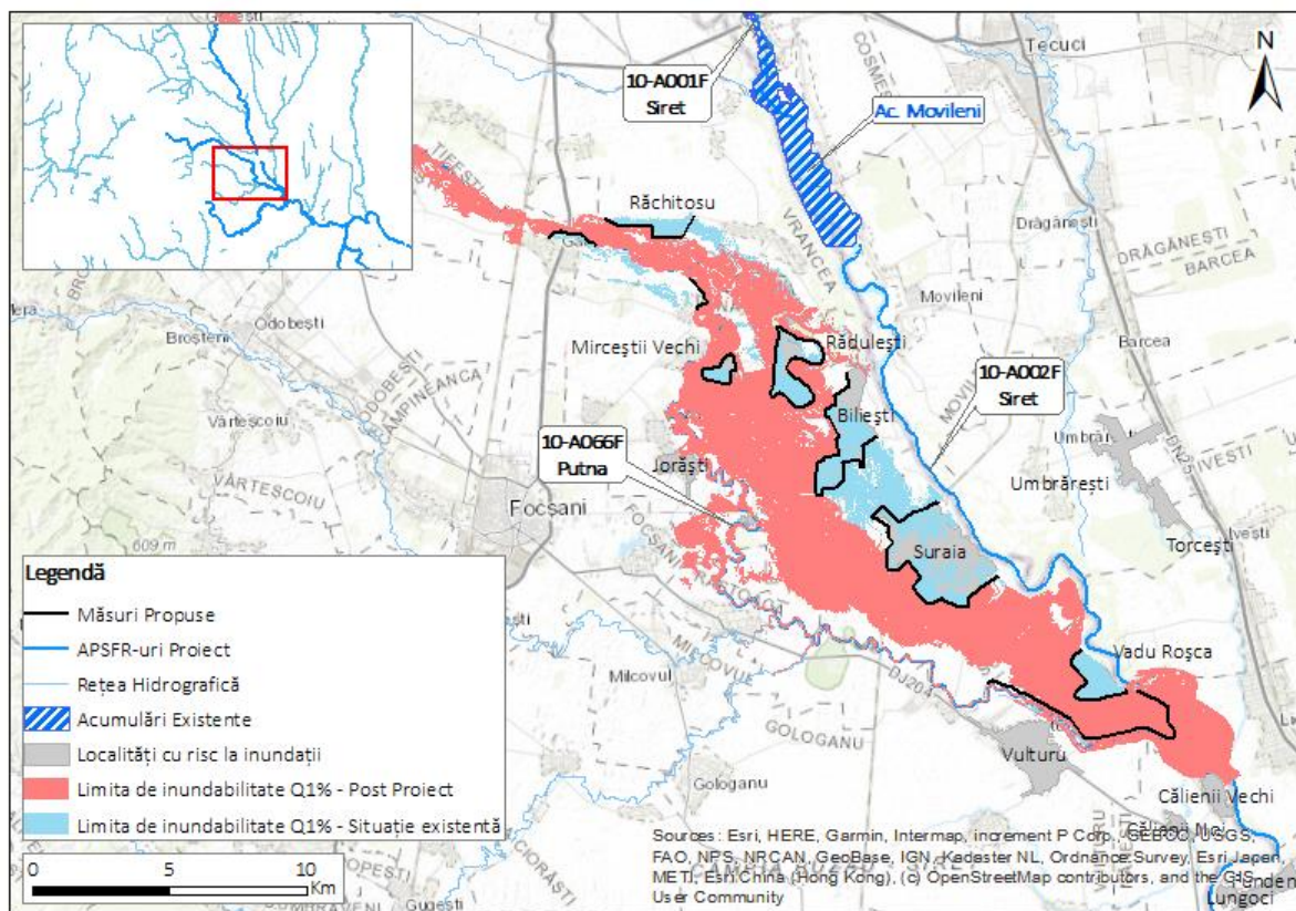
Figura 9: Limita de inundabilitate pre și post implementare proiect Q1%, r. Putna
