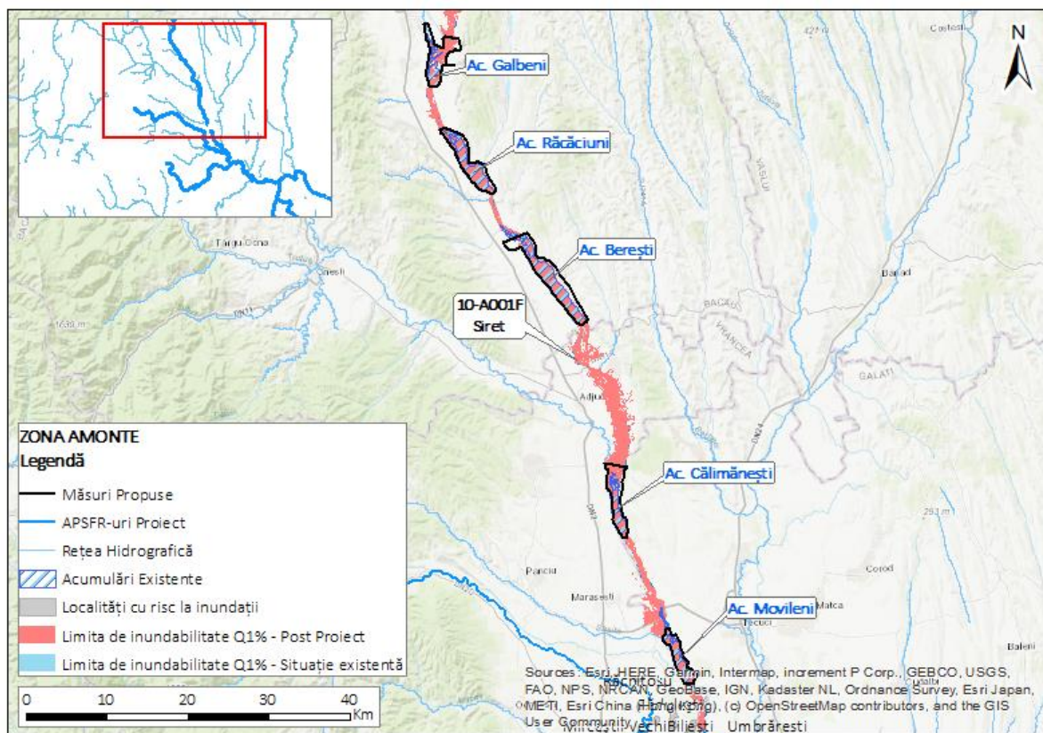
Figura 7a: Zona amonte.Limita de inundabilitate pre și post implementare proiect Q1%, r. Siret
