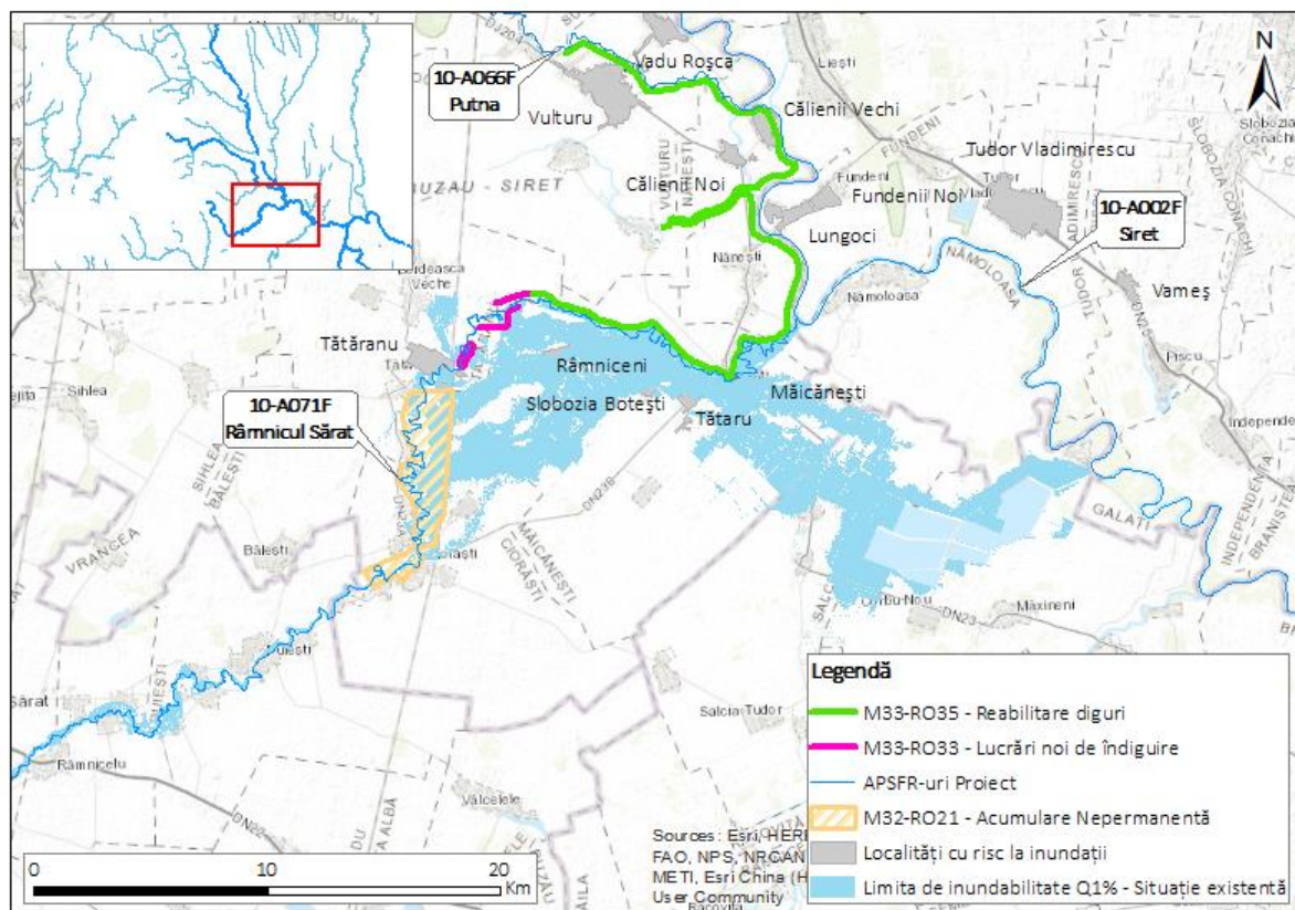
Figura 6: Localizarea măsurilor aferente alternativei preferate și limita de inundabilitate pentru probabilitatea de 1% în situația actuală, r. Râmnicul Sărat
