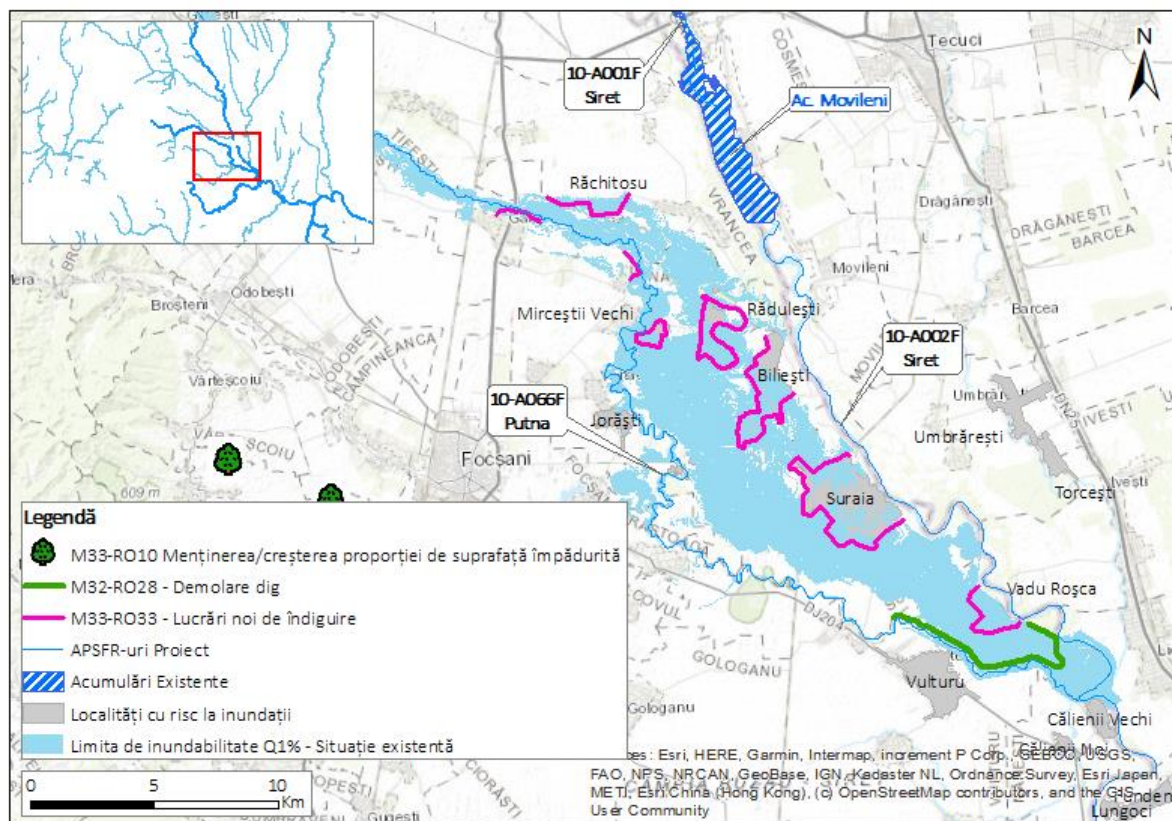
Figura 4b: Zona aval. Localizarea măsurilor aferente alternativei preferate și limita de inundabilitate pentru probabilitatea de 1% în situația actuală, r. Siret
