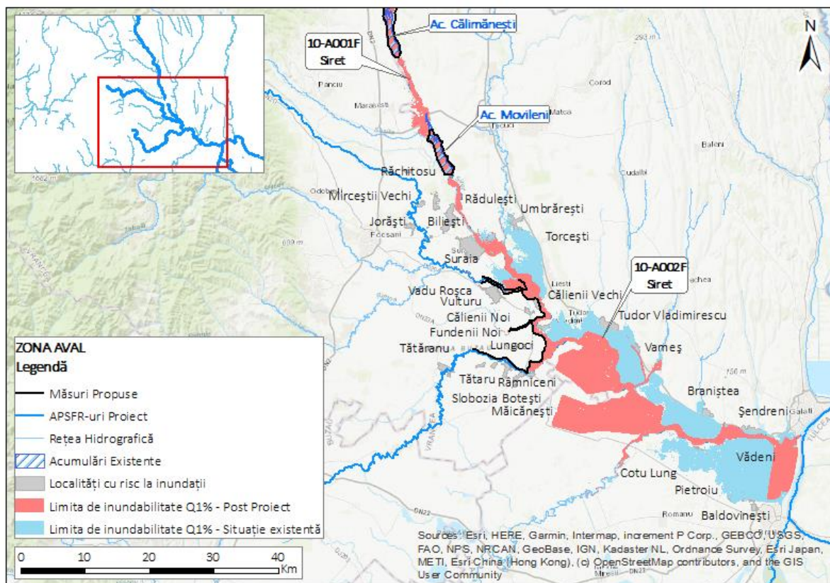
Figura 8b: Zona aval. Limita de inundabilitate pre și post implementare proiect Q1%, r. Siret
