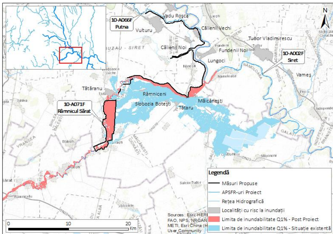
Figura 10: Limita de inundabilitate pre și post implementare proiect Q1%, r. Râmnicul Sărat
